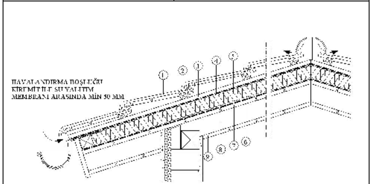
4- ÇATI ARASI KULLANILAN KIRMA ÇATILAR ( ISI YALITIMI MERTEK VEYA ÇATI TAHTASI ÜZERİNDE)
