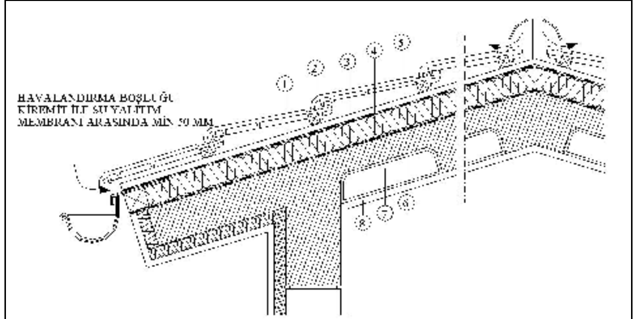
3- ÇATI ARASI KULLANILAN KIRMA ÇATILAR ( BETONARME PLAK VEYA ASMOLEN DÖŞEME VEYA GAZBETON ÇATI PANELİ ÜZERİ)
